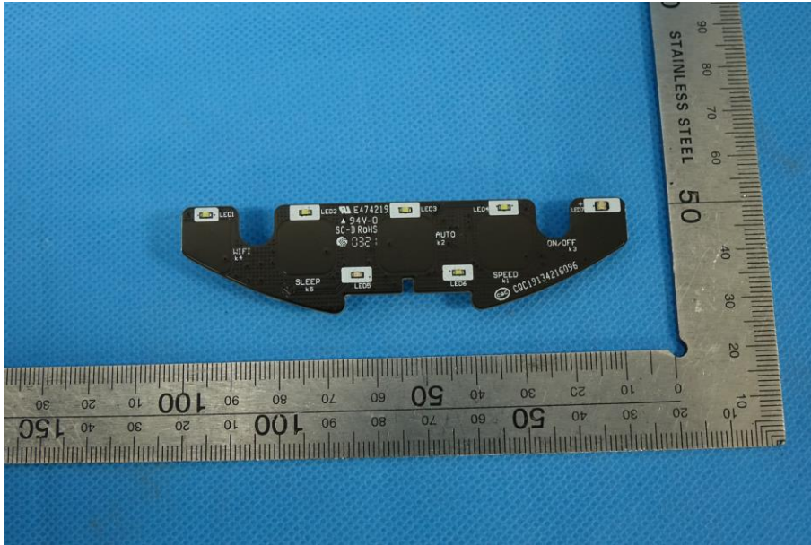
控制电路板背面
