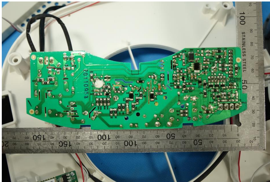
主电路板背面
