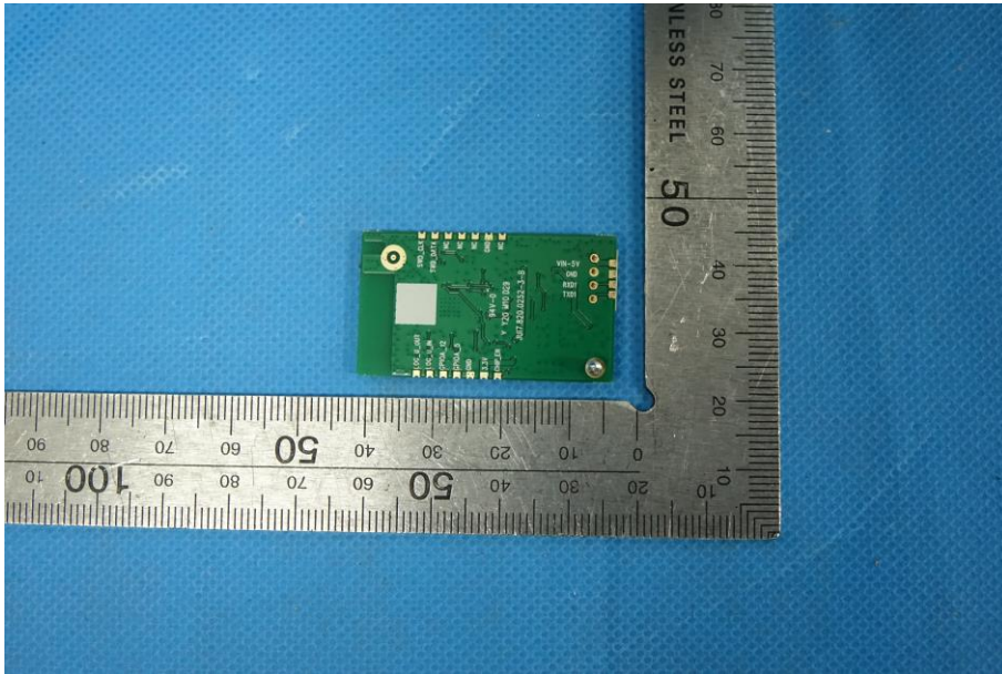
无线模块背面
