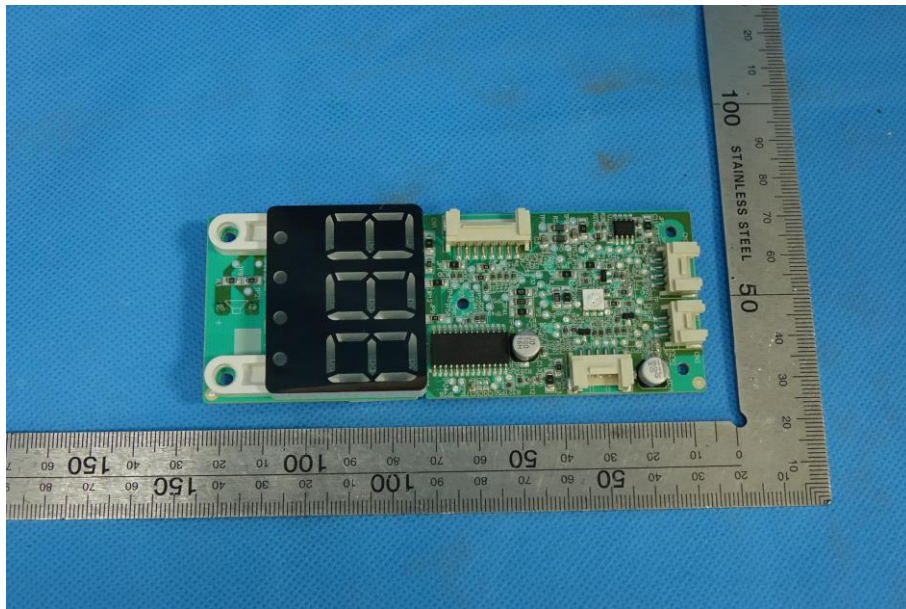
显示电路板正面
