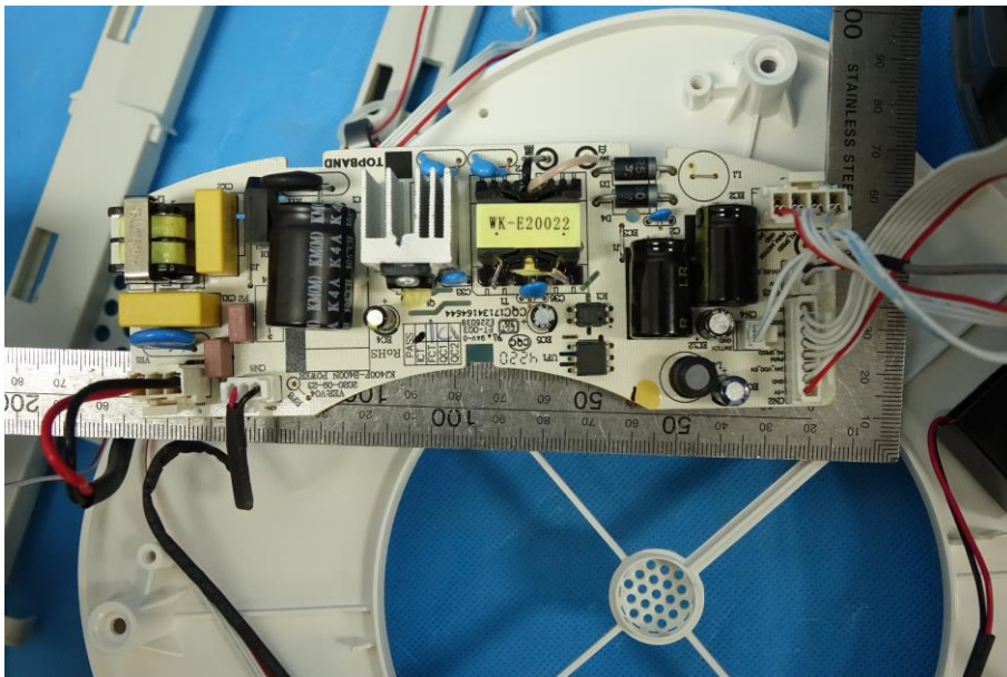
主电路板正面
