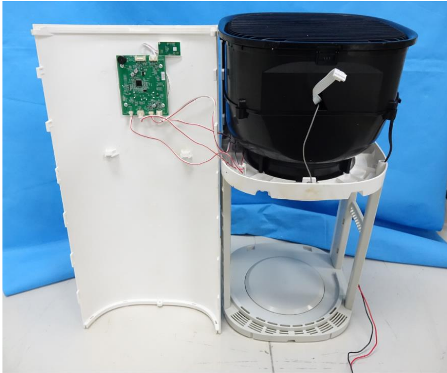
内部结构
