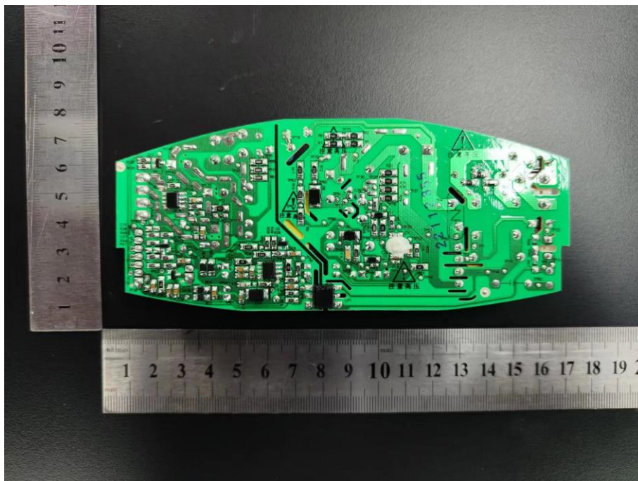
电源板背面
