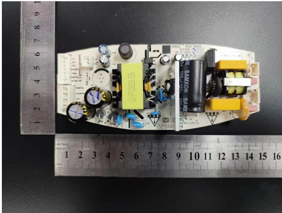
电源板正面
