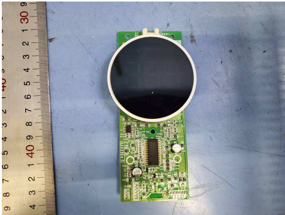
Display PCB
