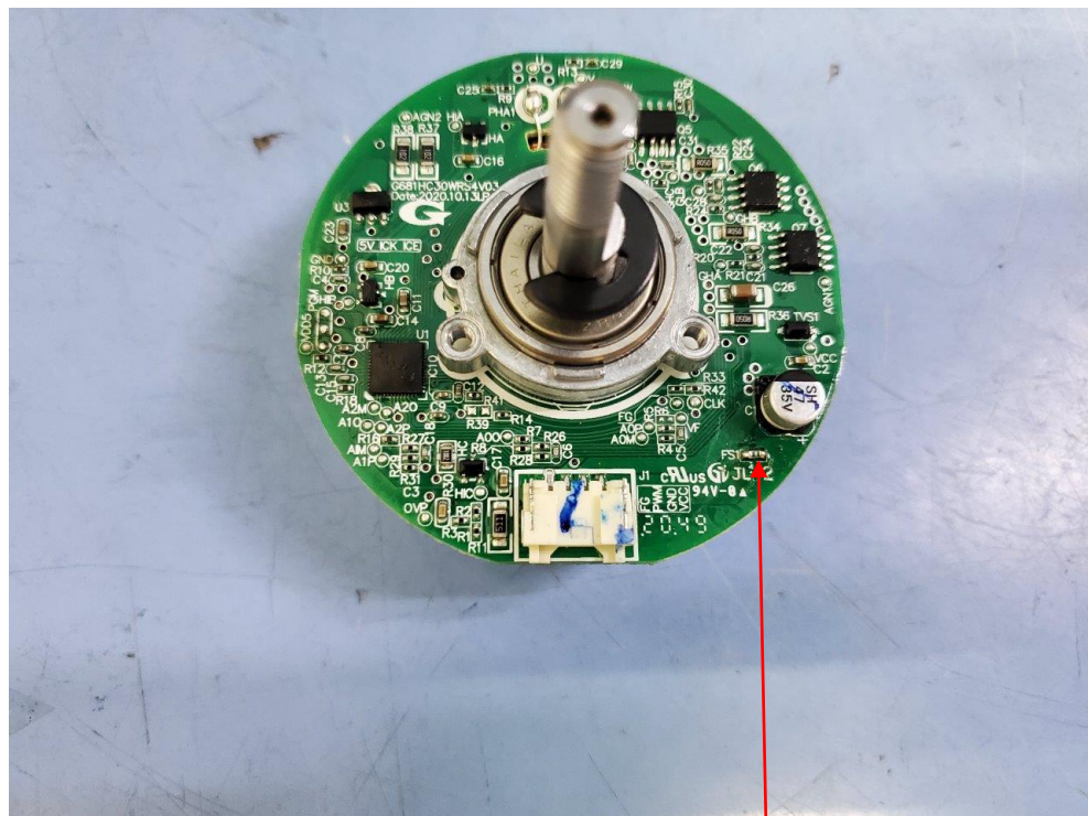
PCB for Fan Motor G0655KHV09, Fuse FS1
