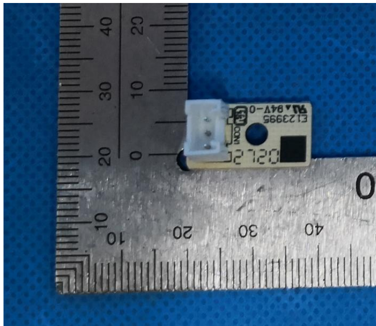
PCB 正面
