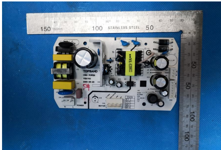
PCB 正面
