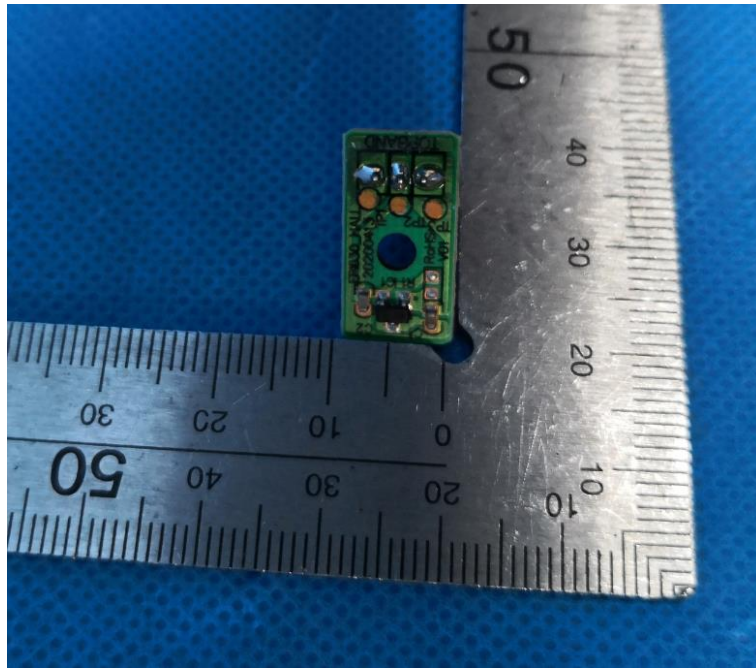
PCB 背面
