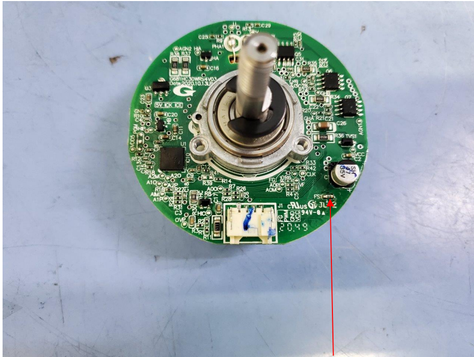
PCB for Fan Motor G0655KHV09, Fuse FS1
