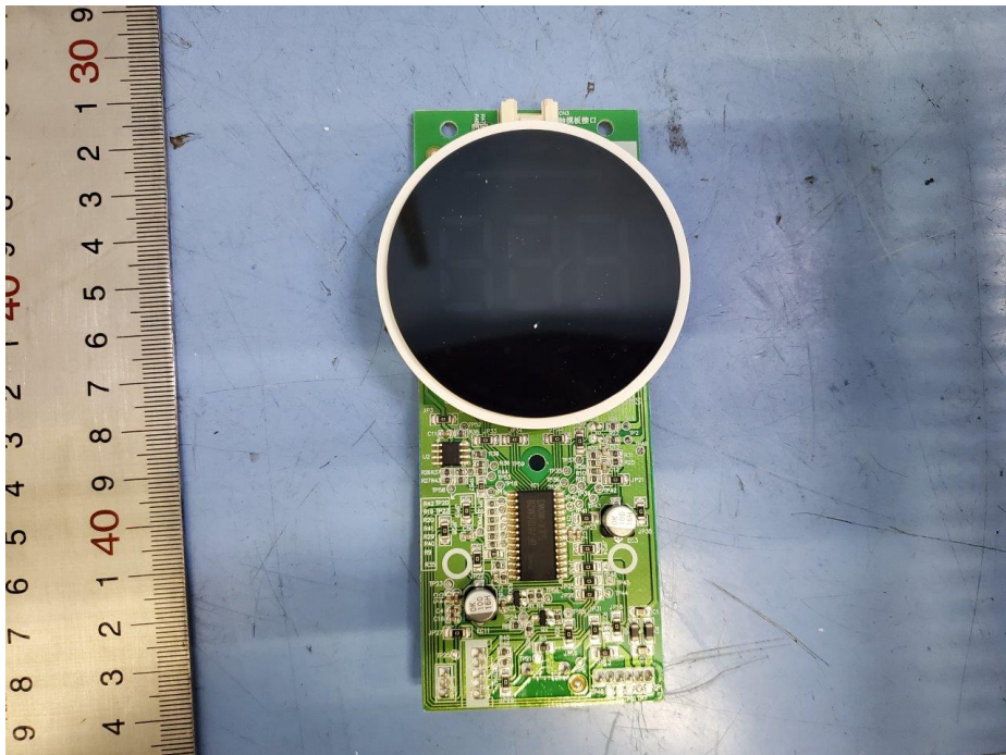
Display PCB
