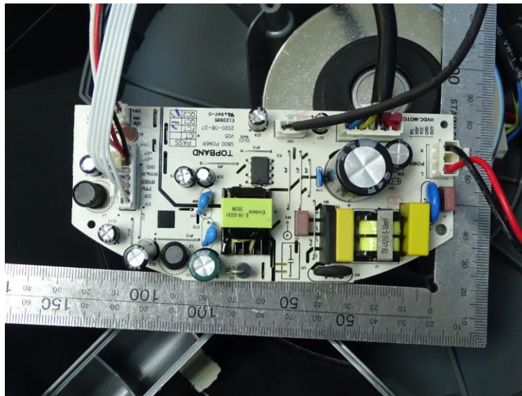
PCB 正面
